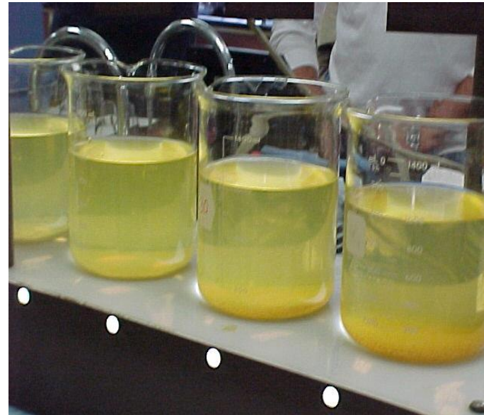
Jar Test
